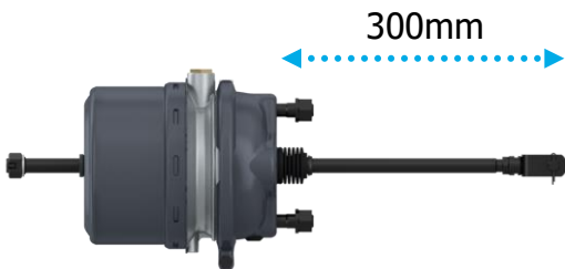
9254910750 SBA 24/75
